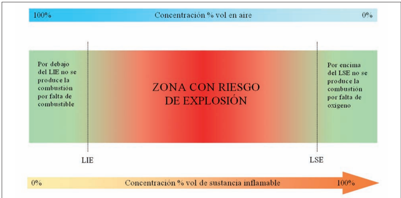
Figura 7 - Rango de explosividad de una sustancia inflamable.
